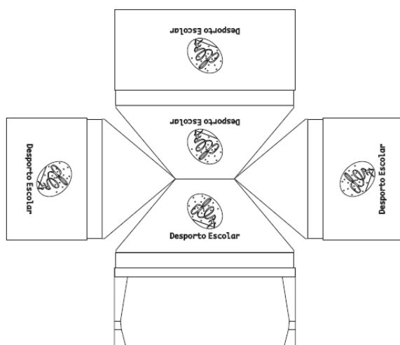
PLANIFICAÇÃO | ESC. 1:100
